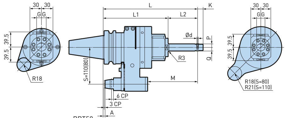
BBT50
