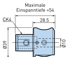
Feinbohrkopf EWN2-22CK4 Verstellbereich 0 - 2mm
