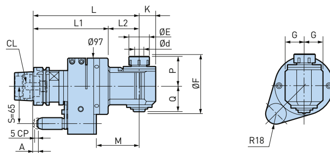
HSK-A63
