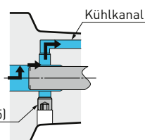
Peripheriekühlung
