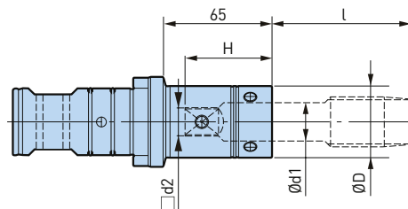
MGT36 (Gewindebohrergrösse JIS: M20 - M36; P1/4, P3/4, P1)
