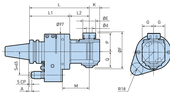
BBT40
