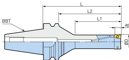
Durchs Zentrum
