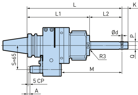
BBT40
