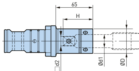
MGT36 (Gewindebohrergrösse DIN: M22 - M36)
