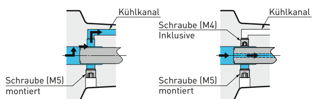
Peripheriekühlung
