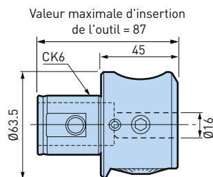
Tête EWN2-54CK6
