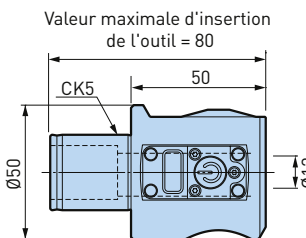
Tête EWE2-32CK5
