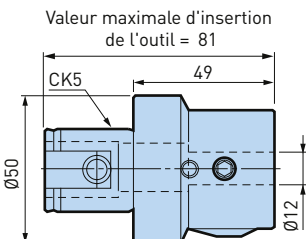
Tête EWB2-32CK5
