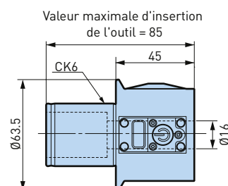
Tête EWE2-54CK6
