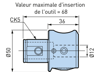
Tête EWN2-32CK5
