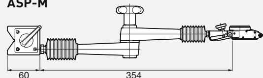
ASP-M
