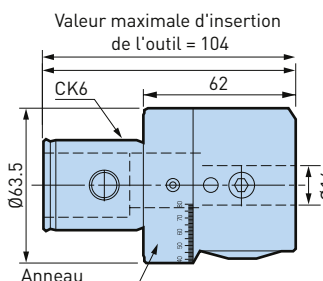
Tête EWB2-50CK6
