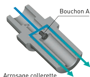
Arrosage collerette
